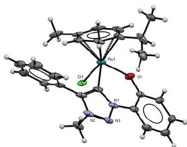
Figura 4. Difracción de rayos X del compuesto 1
